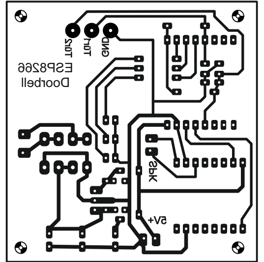
trägerplatine esp8266
