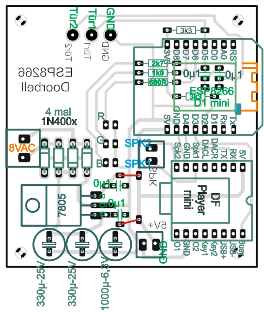
trägerplatine esp8266
