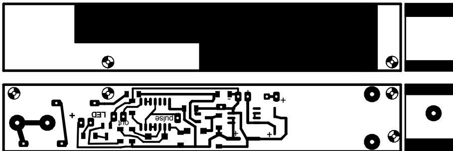
Zählereinheit beide Seiten sind gespiegelt für Kontaktkopie Die Druckseiten werden gegeneinander geklebt und die doppelseitige Platine dazwischengeschoben
