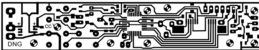
Controllerplatine ist gespiegelt für Kontaktkopie
