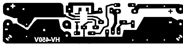
Hochspannungsgenerator für Strahlungsmessgerät
